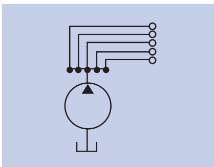
Representación esquemática Sistema Multilínea
