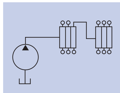
Representación Esquemática Sistema Progresivo
