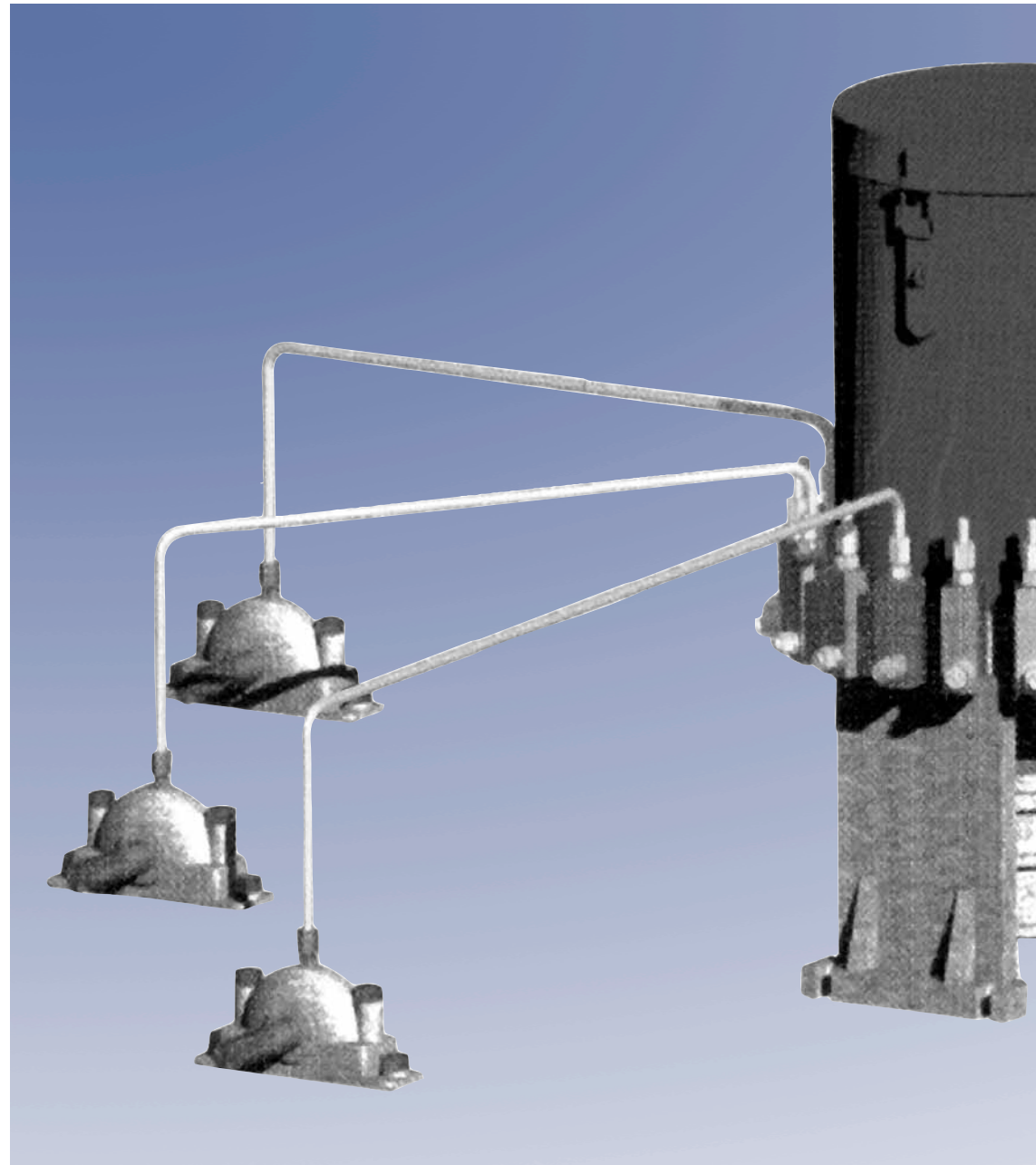
Representación esquemática de Sistema Combinado Multilínea / Progresivo
