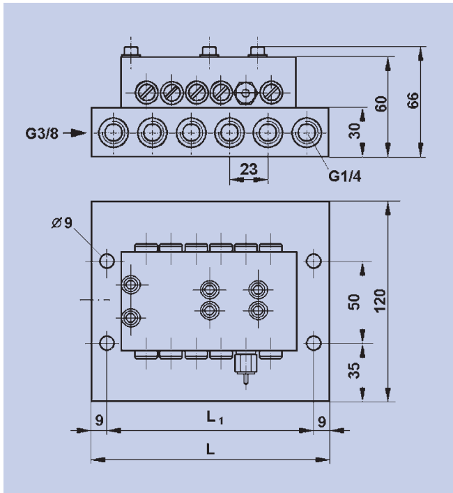
Dimensiones de SSV-FL
